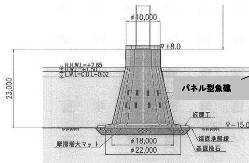
風車基礎部へのパネル型魚礁取付けイメージ
